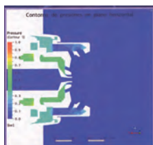
Contorno de presiones plano horizontal
