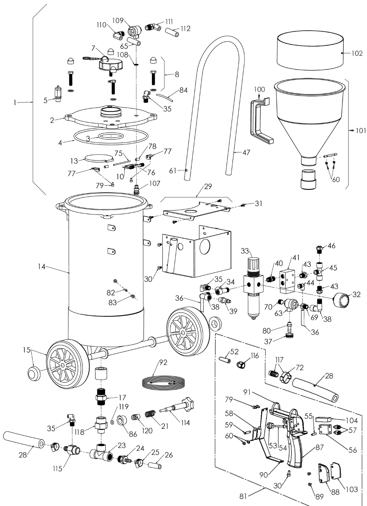
Despiece 2 – Componentes de Repuesto (Arenadora JAFE 10 HD) (Rev.0)
